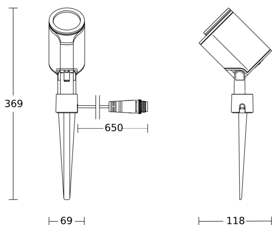
Maßzeichnung 1
